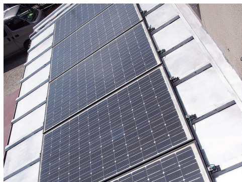
オフグリッドハウス「松江の家」 の太陽光発電パネル
